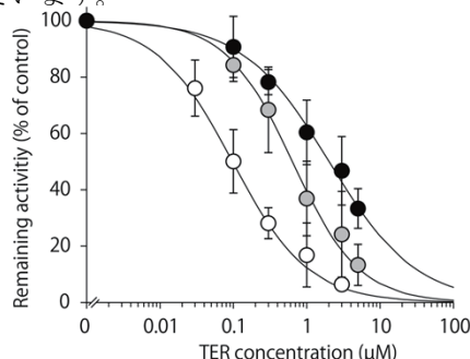
図. CYP2D6 各遺伝的バリエーションの活性に対する阻害剤（テルピナフィン; TER）の阻害特性の差異。 ○: CYP2D6.1, ●: CYP2D6.2, ●: CYP2D6.10 ( Drug Metabol Pharmacokinet 30:321-4, 2015)
