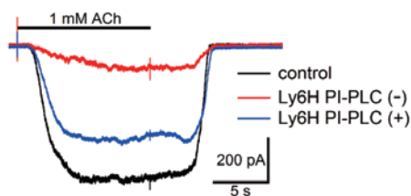
図1: Ly6HのAChに対する \alpha 7 -nAChRの応答電流抑制効果 \alpha 7 -nAChRへのACh投与時に観察される応答電流 (—) とLy6Hの共発現時に観察される応答電流 (—)。Ly6HはGPIアンカー型の膜タンパクであるため、ホスファチジルイノシトール特異的ホスホリラーゼC (PI-PLC) 処理により、Ly6HのAChに対する \alpha 7 -nAChRの応答電流抑制効果は解除される (—)。
