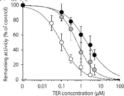
図. CYP2D6 各遺伝的バリエーションの活性に対する阻害剤（テルビナフィン；TER）の阻害特性の差異。 ○：CYP2D6.1，●：CYP2D6.2，●：CYP2D6.10 ( Drug Metabol Pharmacokin 30 :321-4, 2015)
